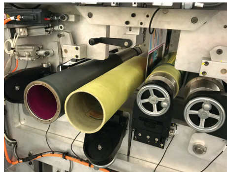
Schnellwechselsystem für Anilox- und Auftragshülse
